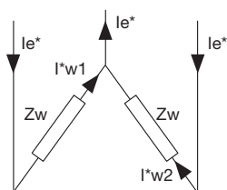
Funcionamiento con falta de un devanado
